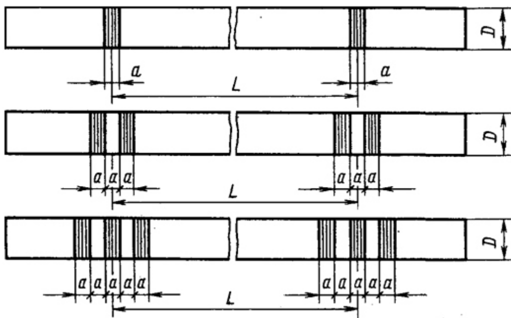
Схема нанесения предупреждающих колец
